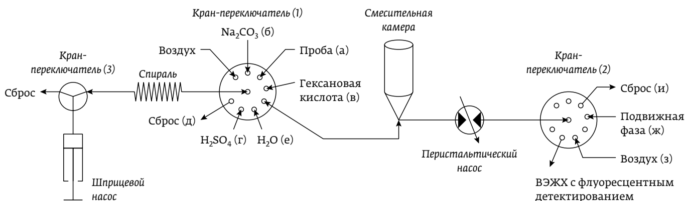
Рис. 1. Гидравлическая схема для автоматизированного определения офлоксацина в гомогенных растворах
